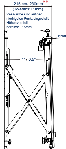
SEITENANSICHT AUSGEFAHREN
