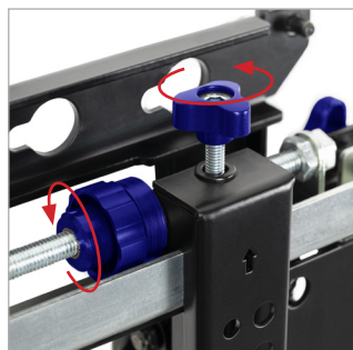
8 Punkte Feinjustage für Tiefe, Höhe und seitliche Bildschirmverstellung
