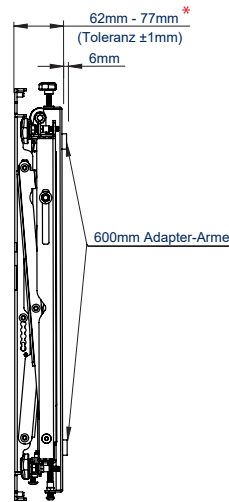
SEITENANSICHT GSCHLOSSEN
